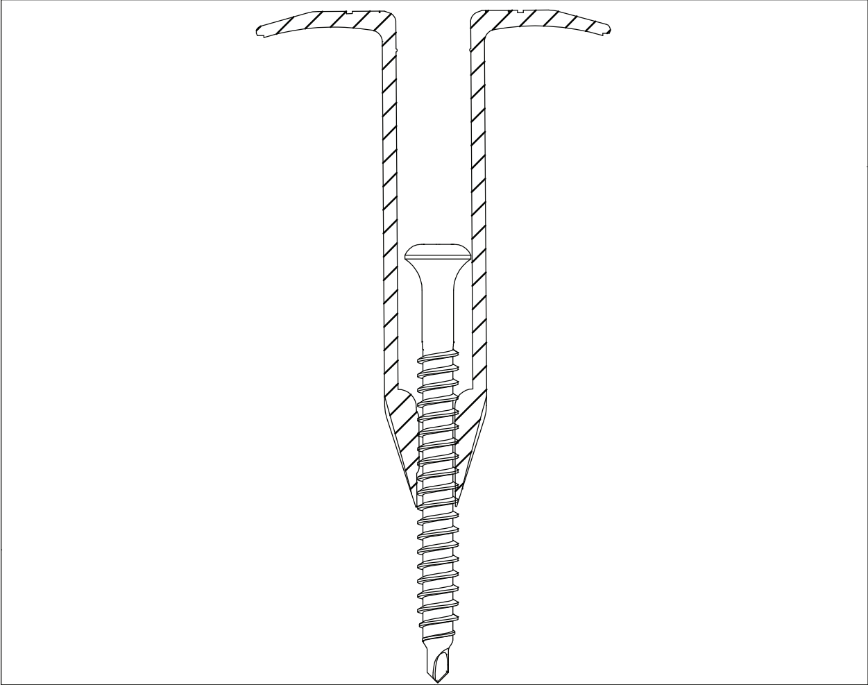
Eurofast EDS-B 5,5 x L
