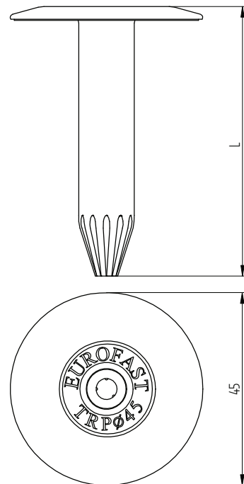
Eurofast TLK- 45
