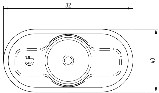
Eurofast DVPEFZK8240D
