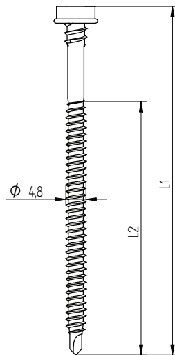
Eurofast EDS-BZTR 4,8 x L
