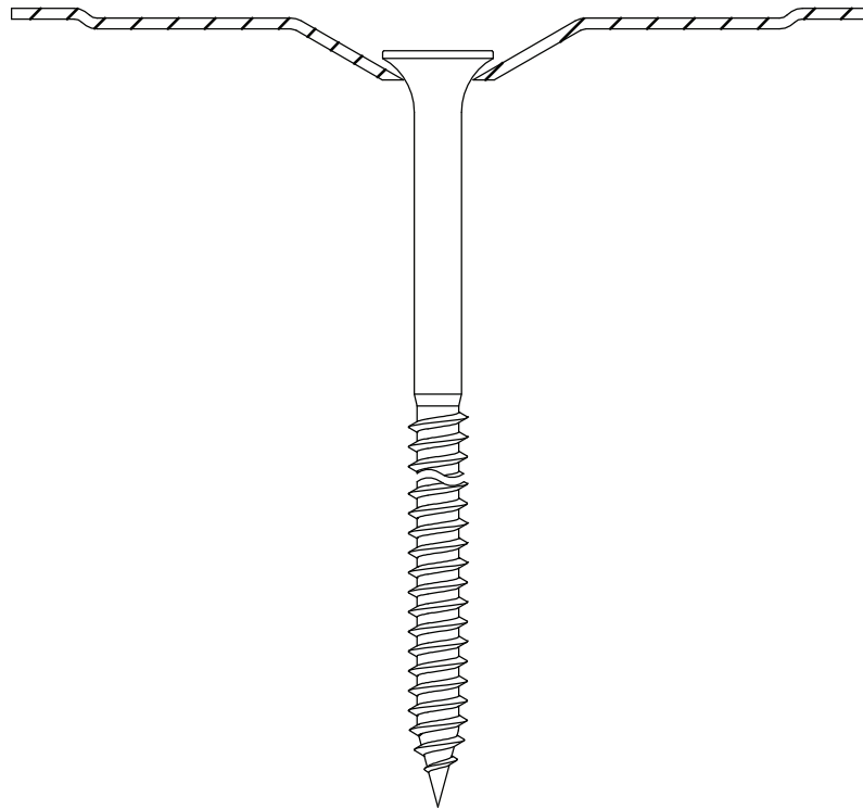
Eurofast EDS-S 4,8 x L
