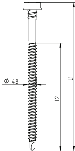
Eurofast EDS-BZT 4,8 x L
