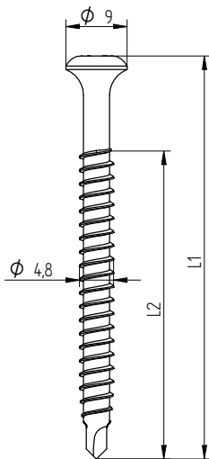
Eurofast EDS-SRB 4,8 x L
