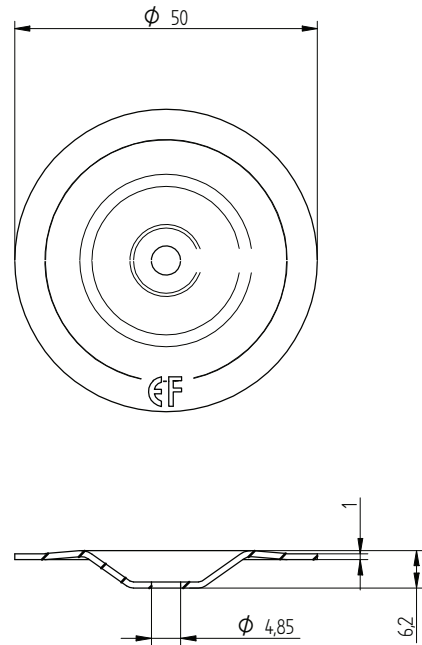
Eurofast DVP-EF-5010DFR
