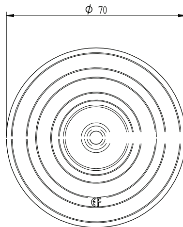
Eurofast DVP-EF-7005N
