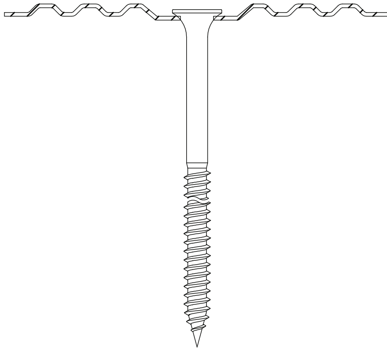
Eurofast EDS-S 4,8 x L
