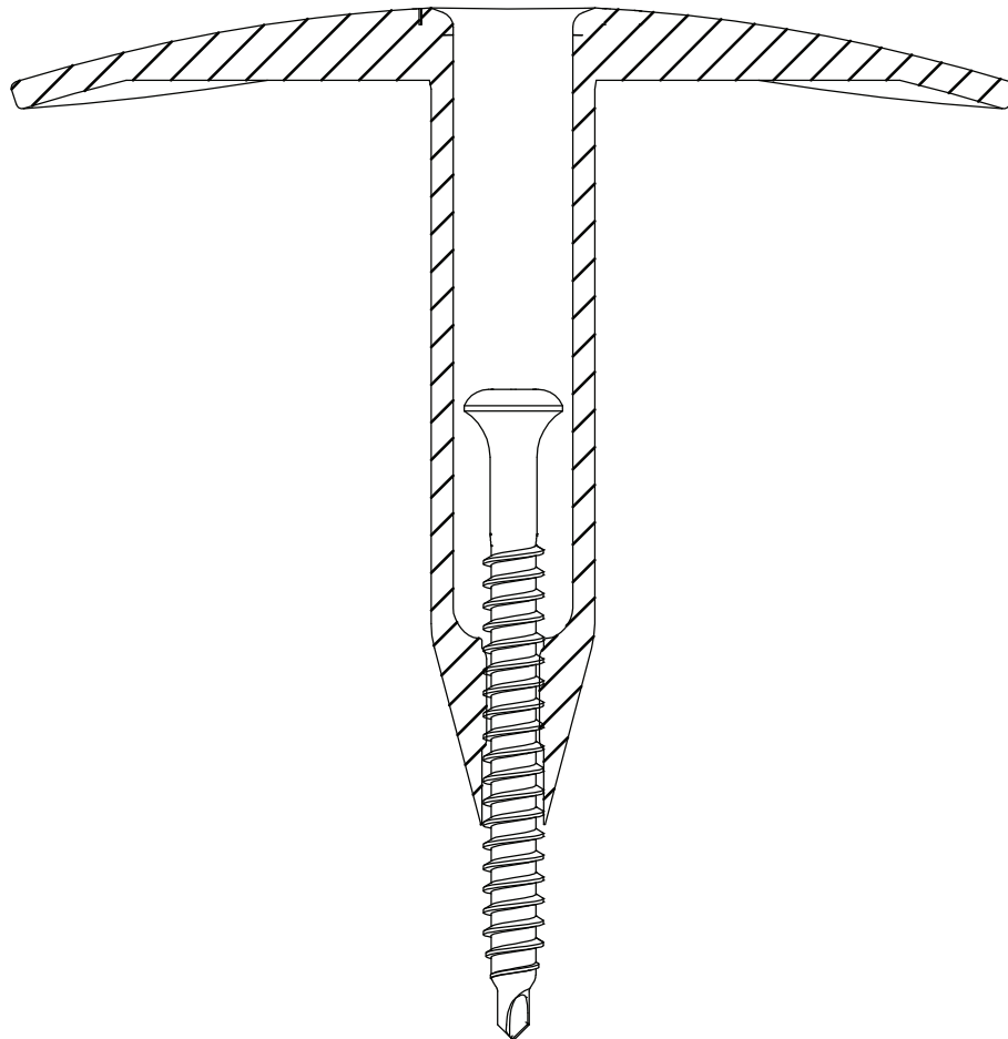
Eurofast TWP-8040
