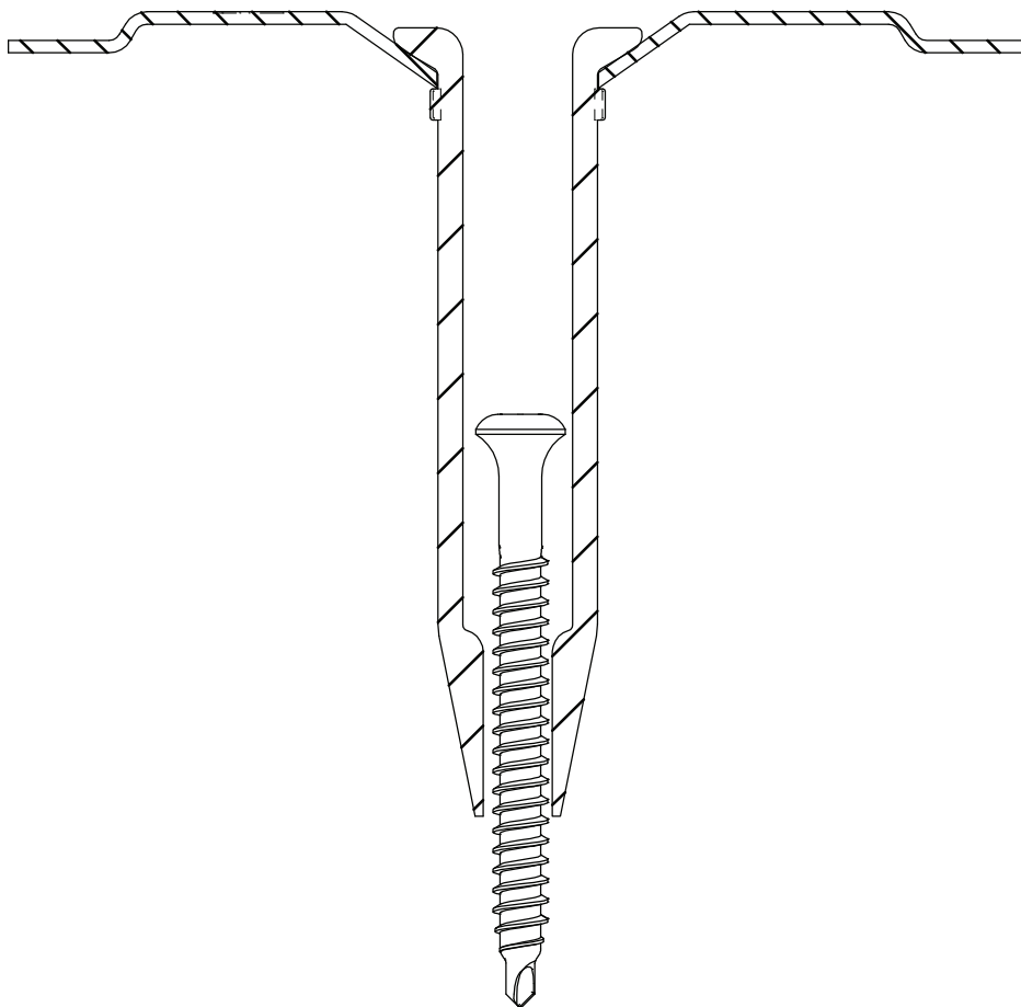
Eurofast KMT-15 Eurofast DVPKMT-8240D
