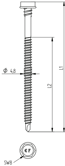
Eurofast EDS-BZTR/BGTR 4,8 x L
