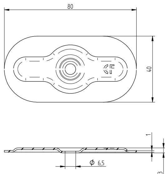
Eurofast DVP-EF-8040 N
