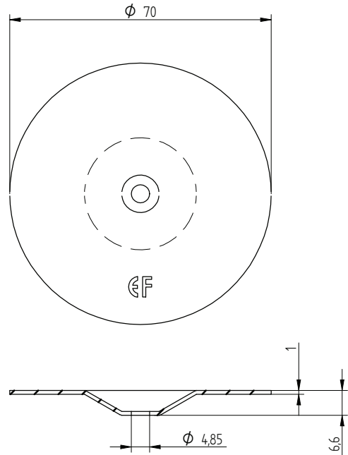
Eurofast DVP-EF-7010DFR
