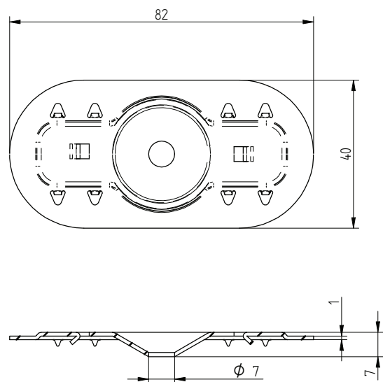
Eurofast DVP-DFB8240D
