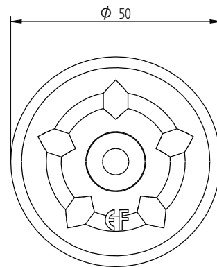
Eurofast DVP-EF-5010N
