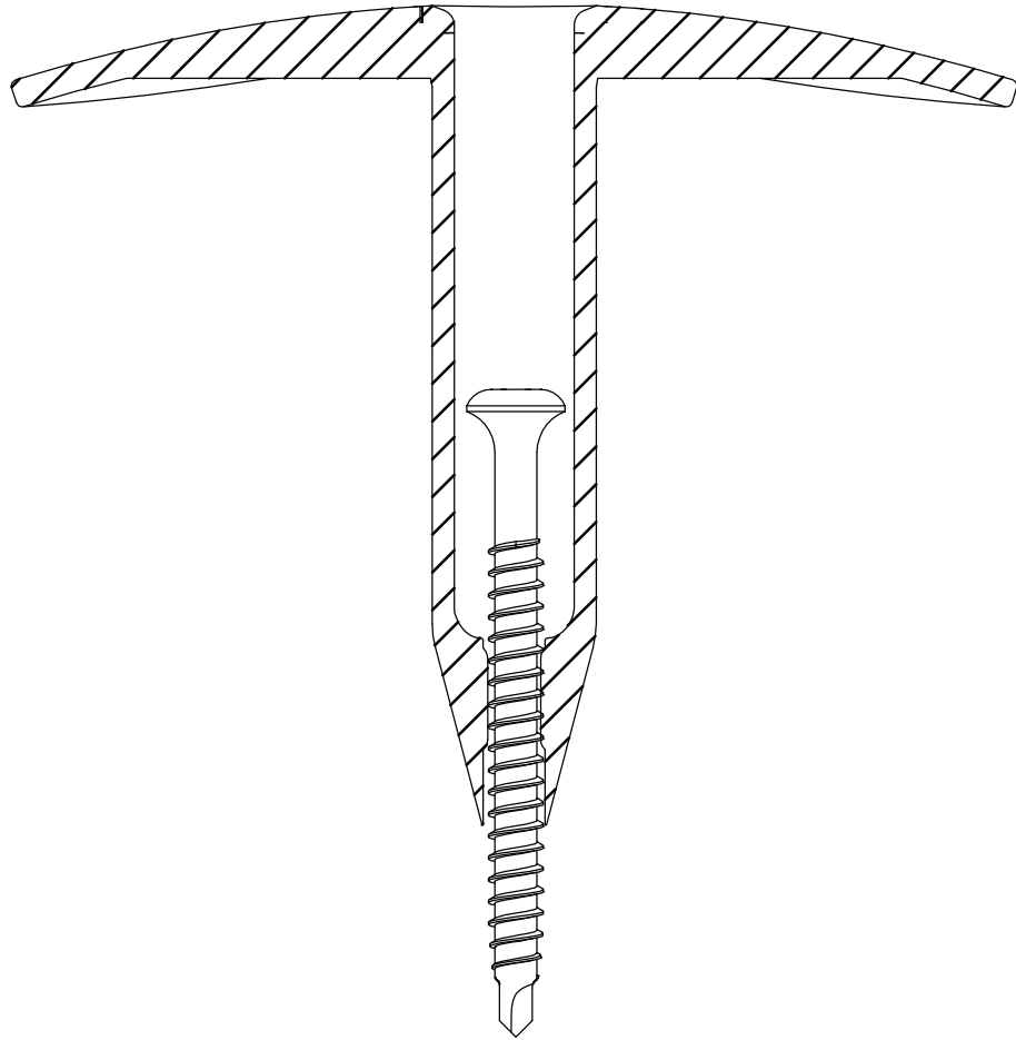
Eurofast TWP-8040
