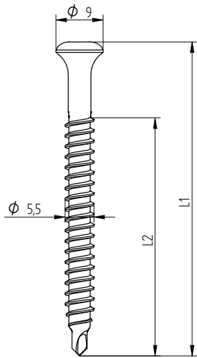
Eurofast EDS-B 5,5 x L
