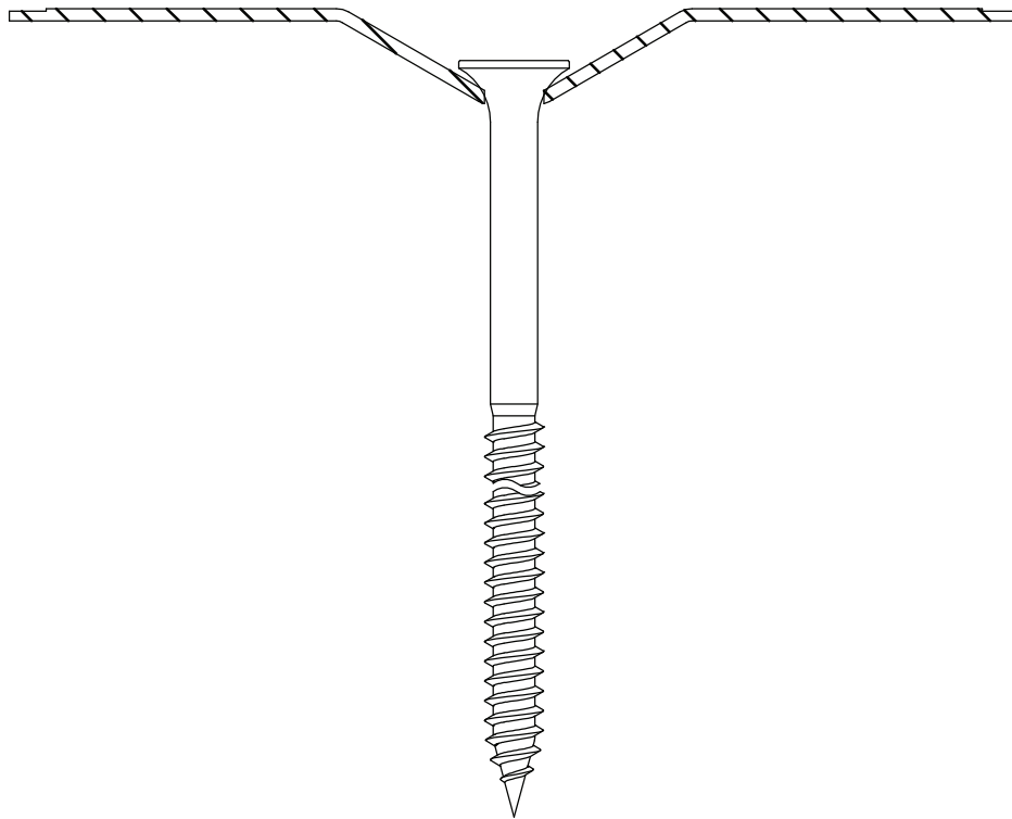
Eurofast EDS-S 4,8 x L
