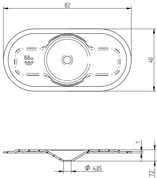
Eurofast DVPEFZK8240D
