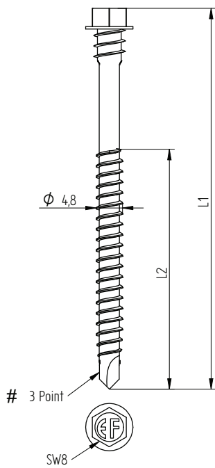
Eurofast EDS-BZTHD/BGTHD 4,8 x L
