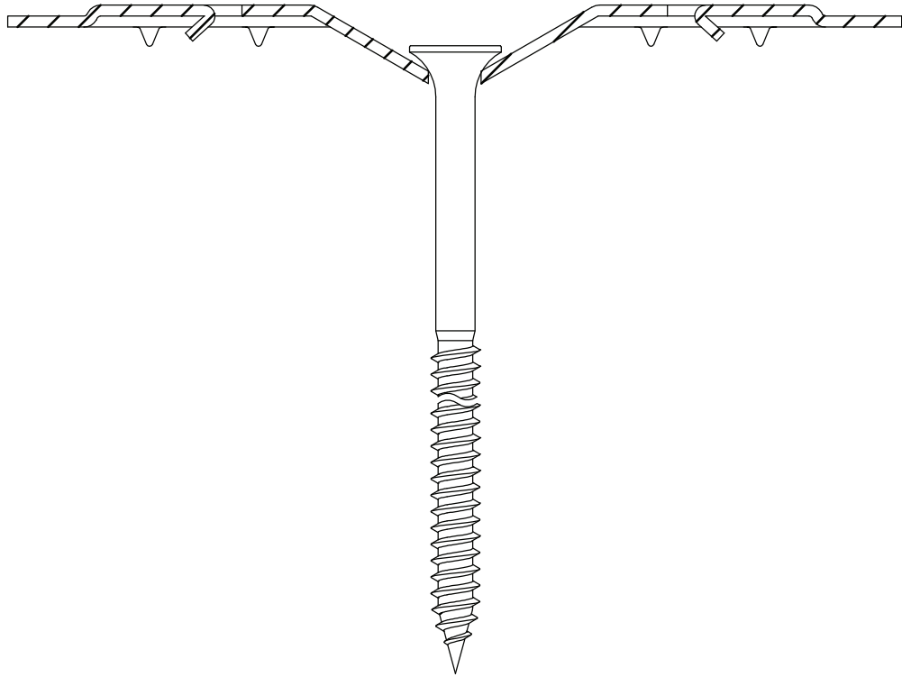
Eurofast EDS-S 4,8 x L
