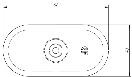
Eurofast DVP-EF-8240XH
