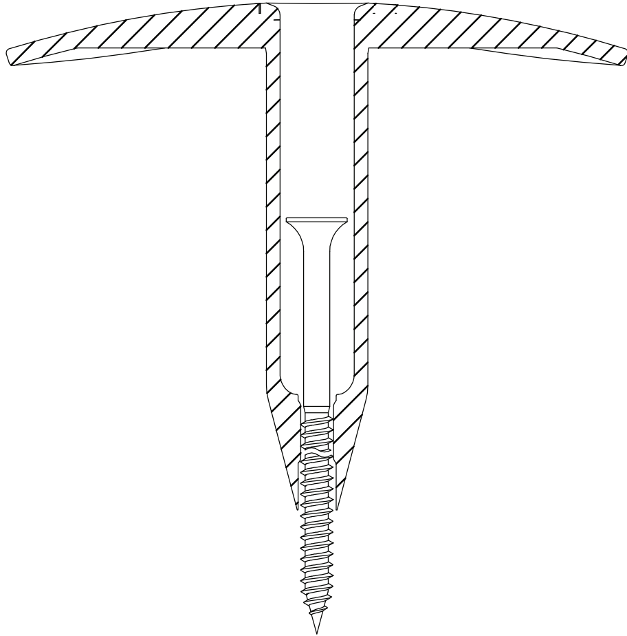
Eurofast EDS-S 4,8 x L
