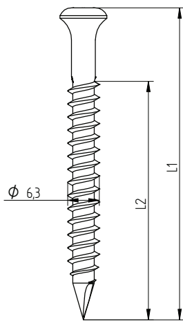
Eurofast EFHD 6,3 x L
