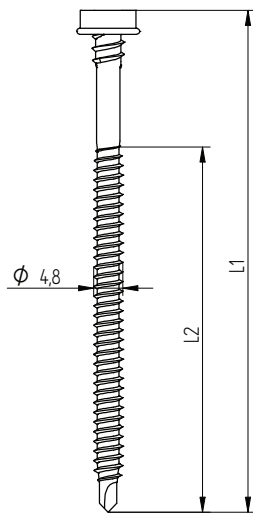
Eurofast EDS-BZTR/BGTR 4,8 x L
