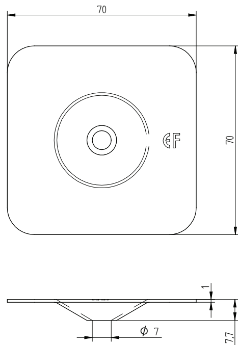
Eurofast DVP-DF-7070D
