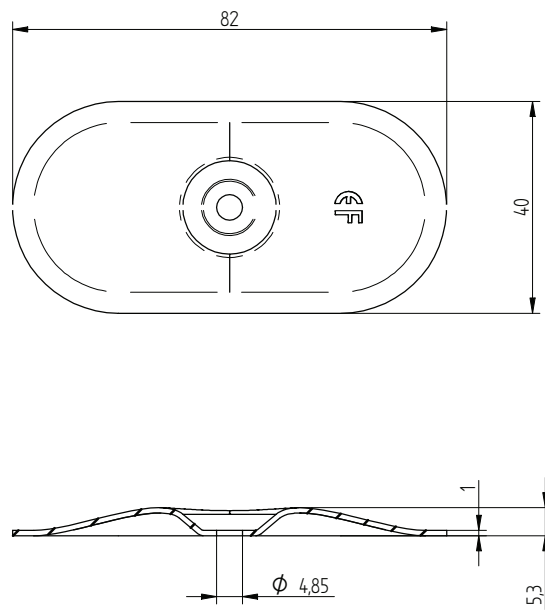
Eurofast DVP-EF-8240XH
