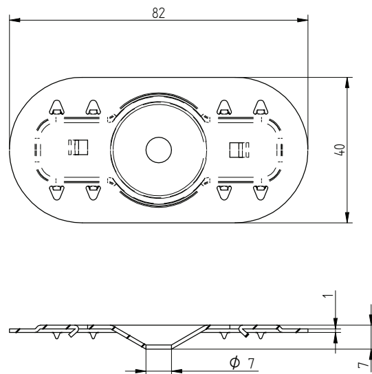
Eurofast DVP-DFB8240D
