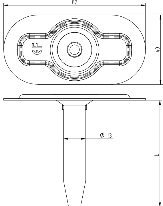
Eurofast KMT-15 Eurofast DVPKMT-8240D 82
