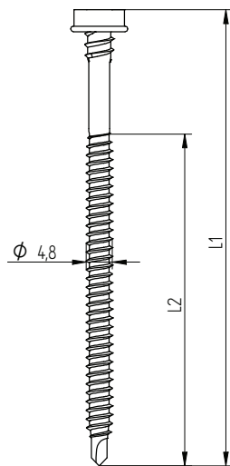
Eurofast EDS-BZT/BGT 4,8 x L
