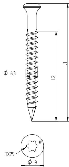
Eurofast EFHD 6,3 x L
