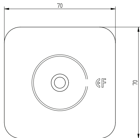
Eurofast DVP-DF-7070D
