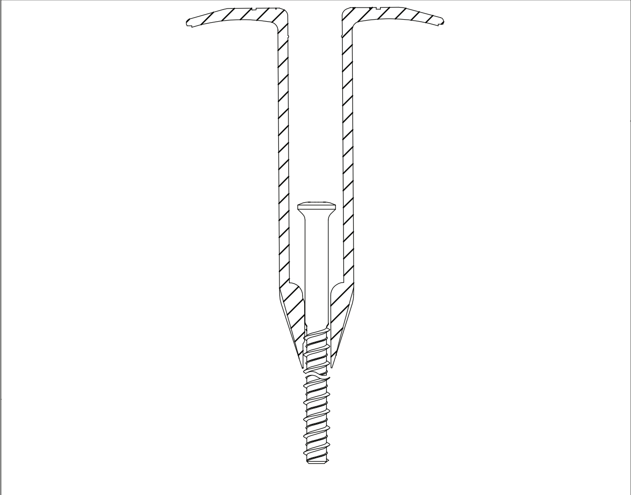
Eurofast EFR 6,3 x L
