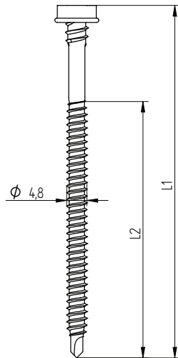
Eurofast EDS-BZT/BGT 4,8 x L
