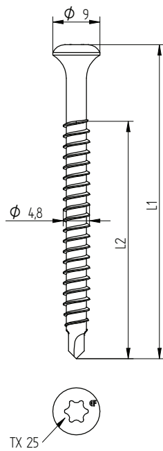
Eurofast EDS-B 4,8 x L
