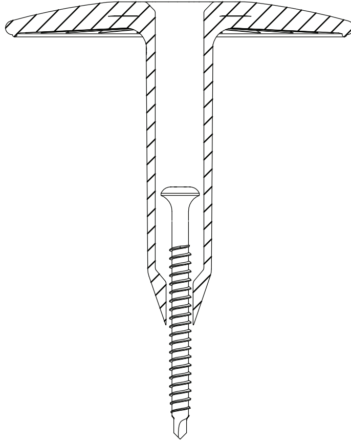
Eurofast EDS-SRB 4,8 x L
