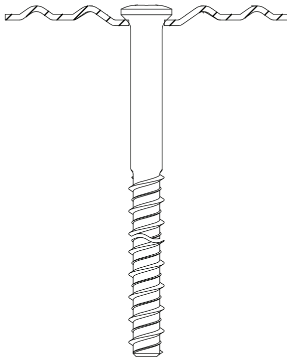
Eurofast DVP-EF-5010N
