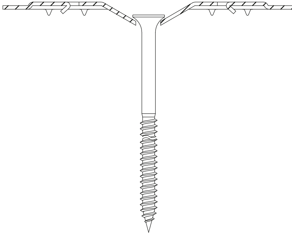
Eurofast EDS-S 4,8 x L
