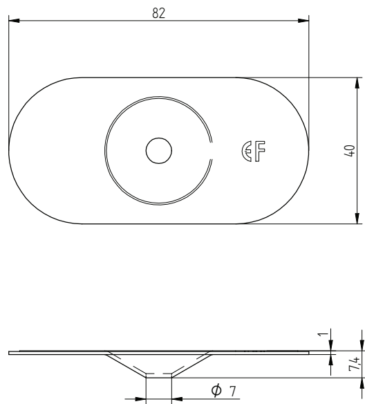
Eurofast DVP-DF-8240D
