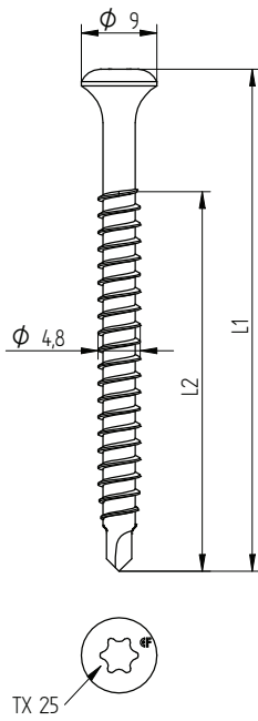
Eurofast EDS-B 4,8 x L
