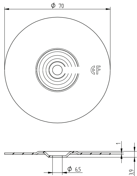
Eurofast DVP-EF-7010N
