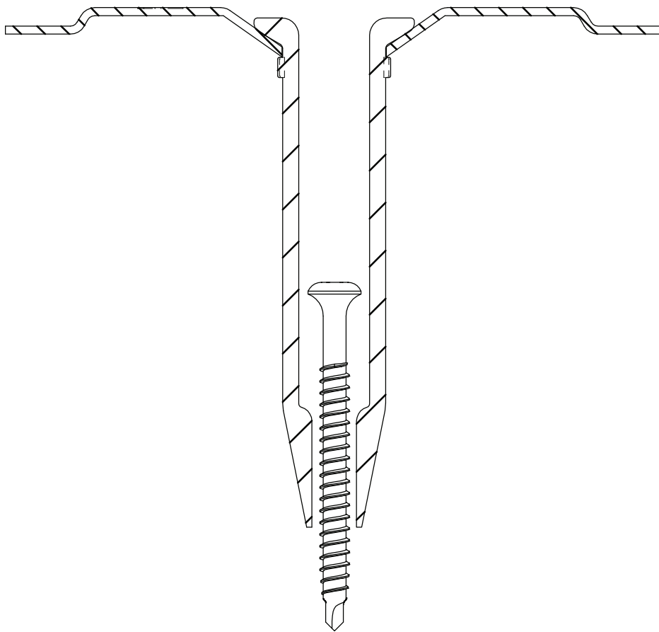
Eurofast KMT-15 Eurofast DVPKMT-8240D
