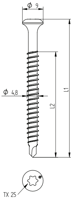
Eurofast EDS-SRB 4,8 x L
