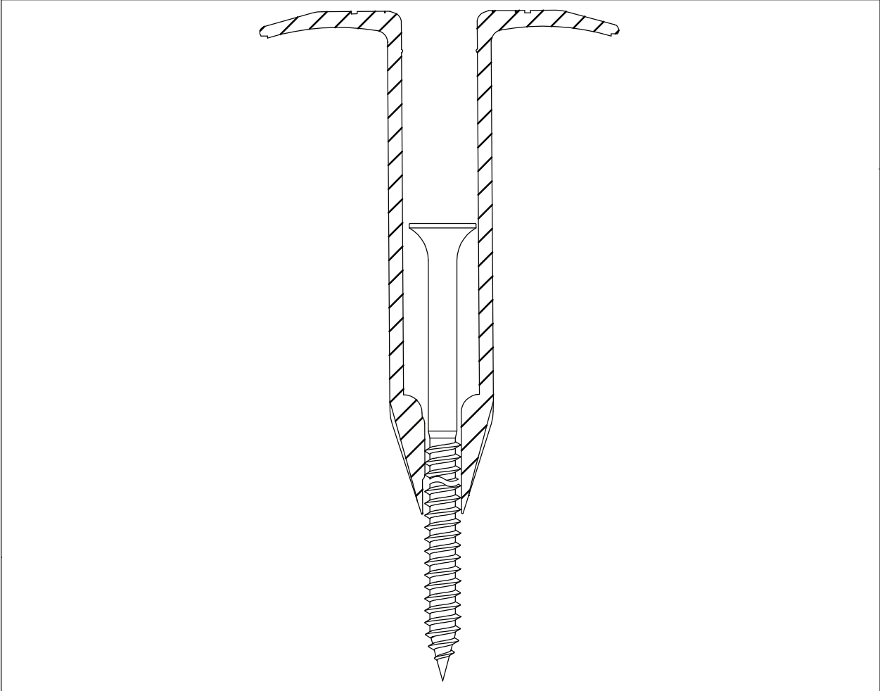
Eurofast EDS-S 4,8 x L
