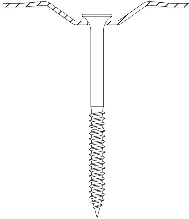
Eurofast EDS-S 4,8 x L
