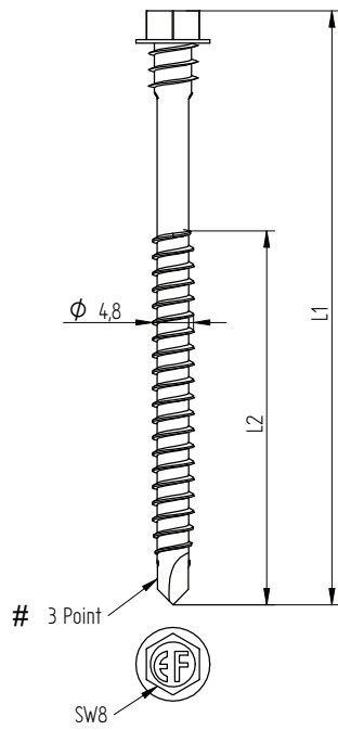
Eurofast EDS-BZTHD 4,8 x L
