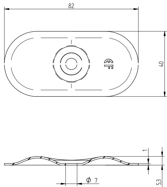
Eurofast DVP-DF8240XH
