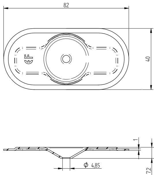
Eurofast DVPEFZK8240D
