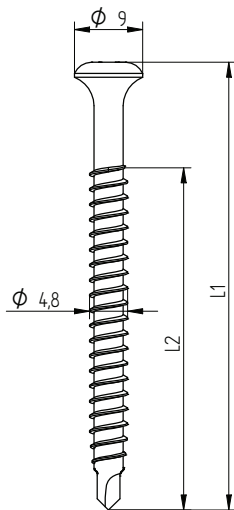
Eurofast EDS-B 4,8 x L
