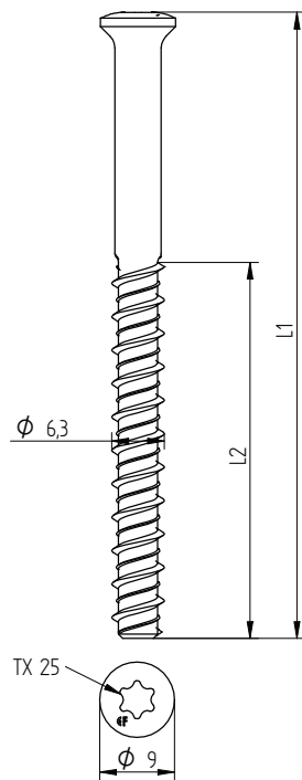
Eurofast EFR 6,3 x L
