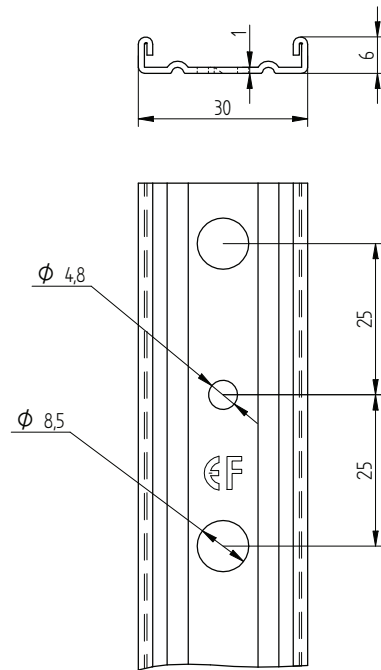
Eurofast EDF-BAR-F
