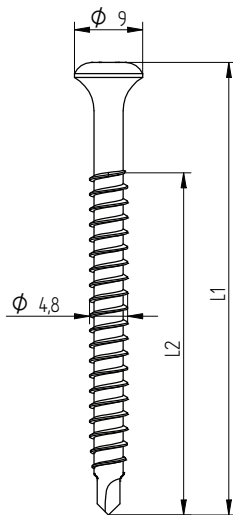
Eurofast EDS-B 4,8 x L
