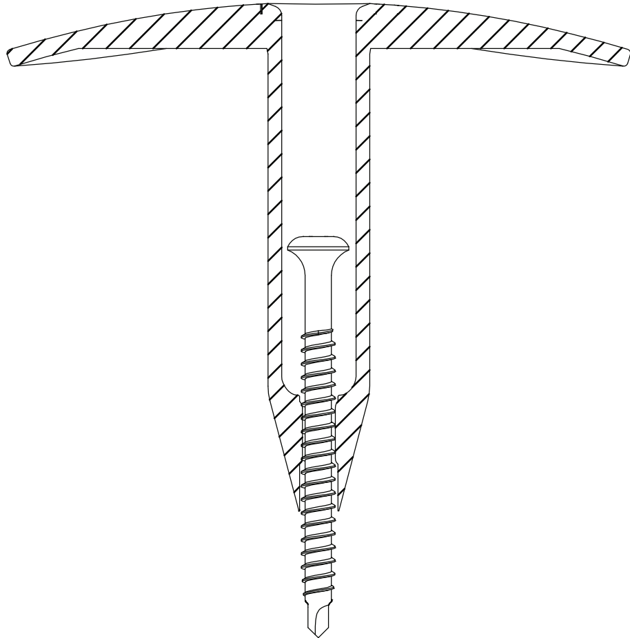
Eurofast EDS-SRB 4,8 x L
