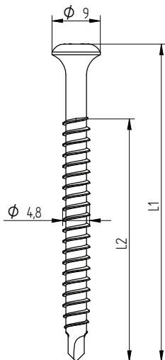
Eurofast EDS-SRB 4,8 x L
