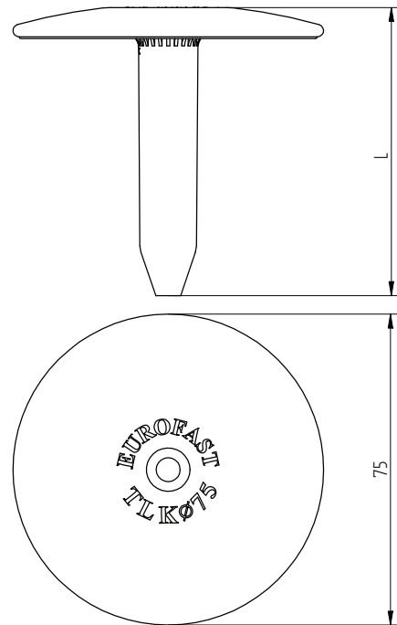
Eurofast TLK-75
