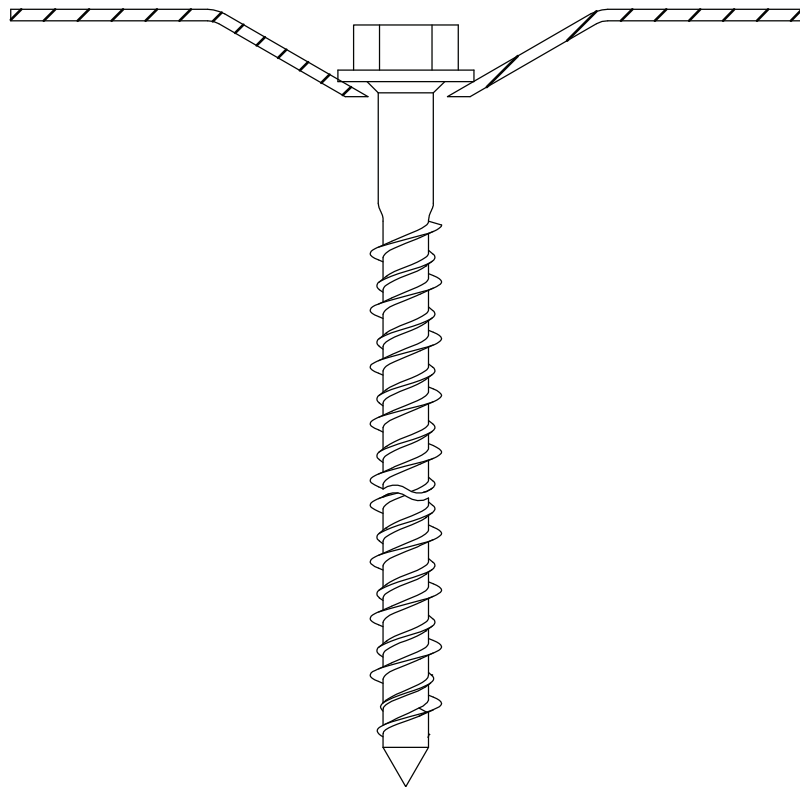
Eurofast DFCF 6,3 x L
