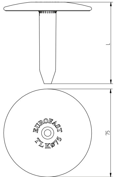
Eurofast TLK-75
