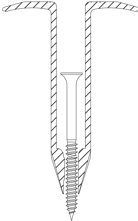
Eurofast EDS-S 4,8 x L
