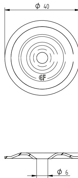
Eurofast DVP-EF-4010N
