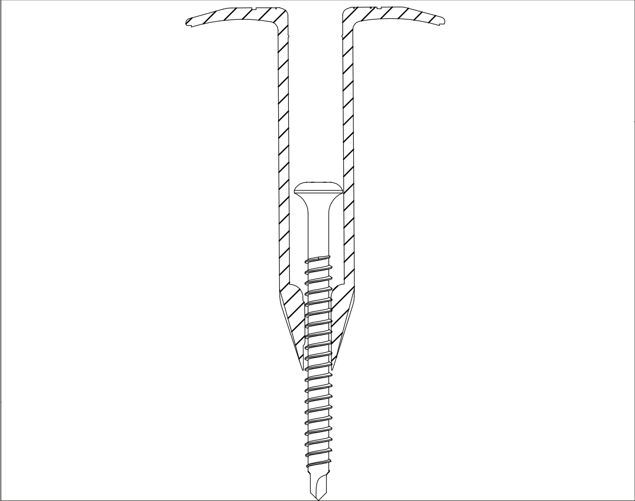
Eurofast EDS-B 4,8 x L
