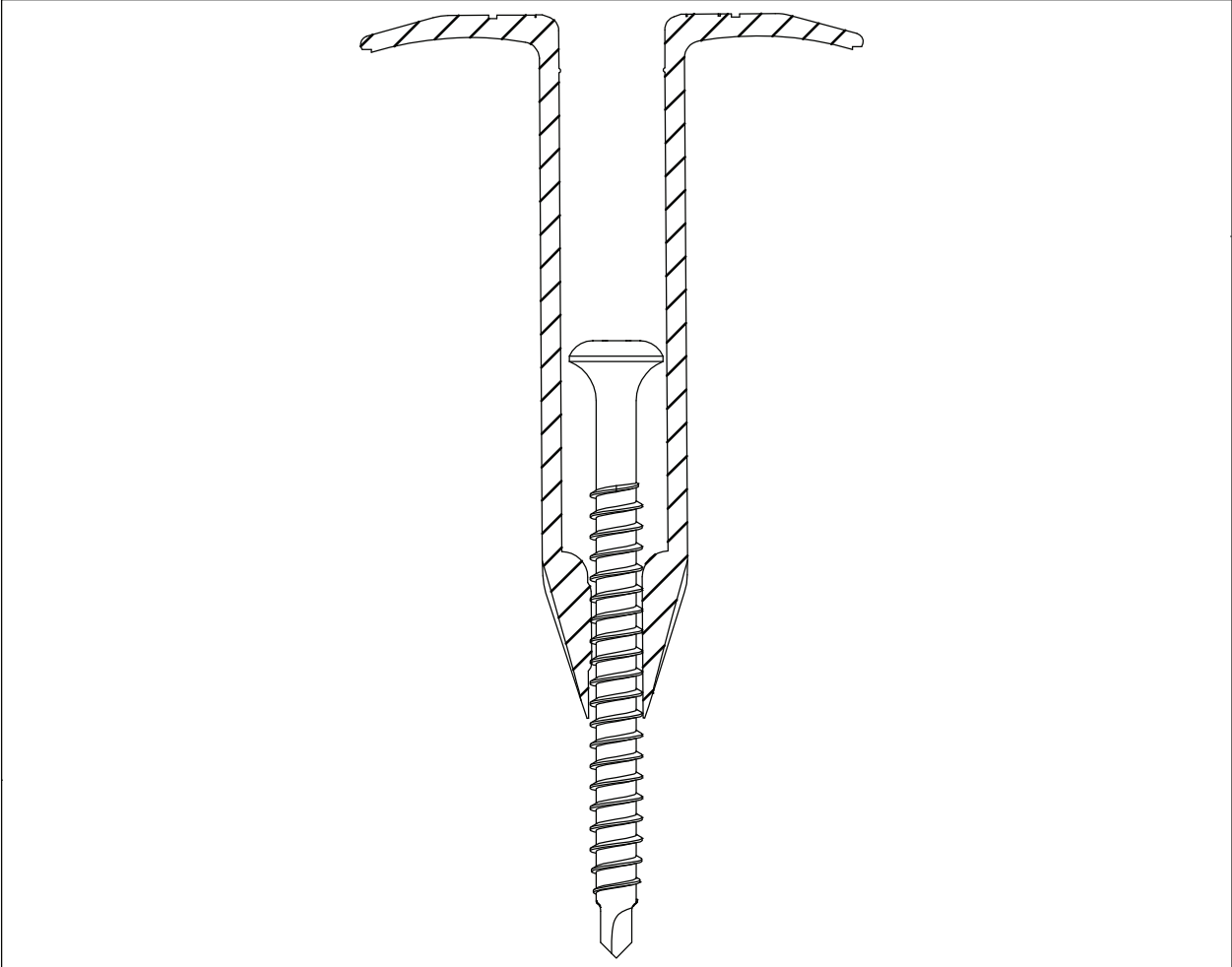
Eurofast EDS-SRB 4,8 x L
