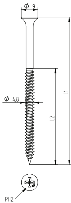
Eurofast EDS-S 4,8 x L
